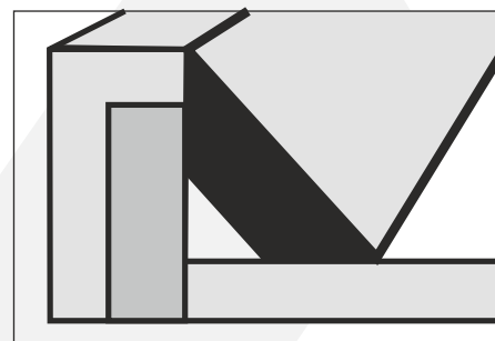
wärme gedämmte Attika WLS 023
